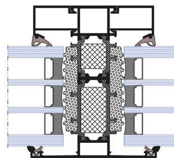
Querschnitt Pfosten Festverglasung
