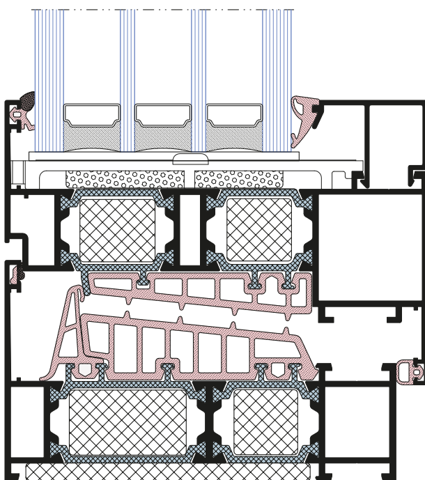
Querschnitt Drehkippfenster
