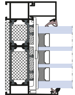
Querschnitt Blendrahmen Festverglasung
